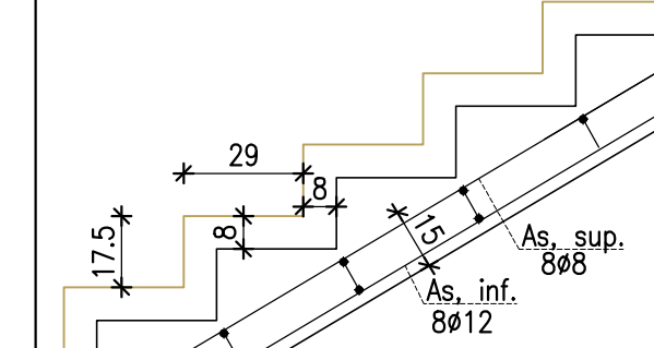
DETTAGLIO GRADINO RAMPA 1-2-3 scala 1:20
