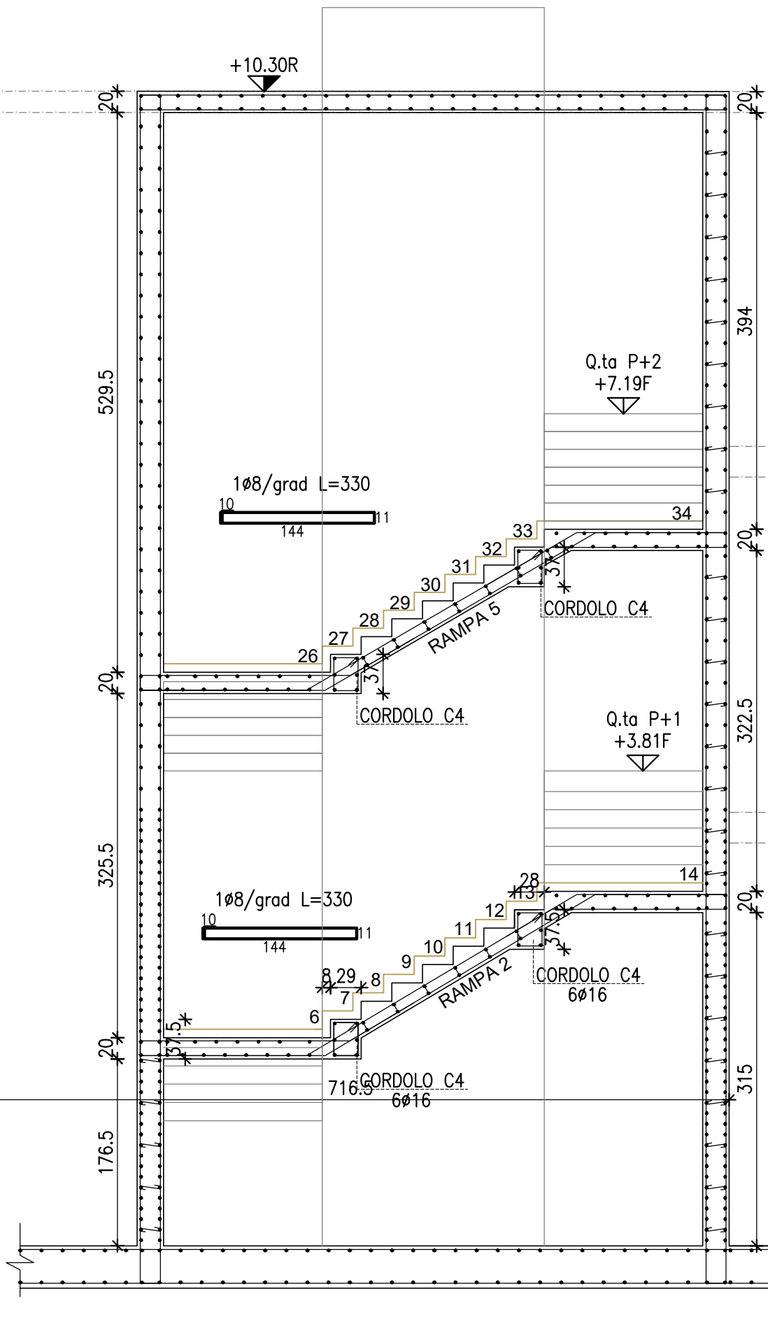
SEZIONE S2 scala 1:50
