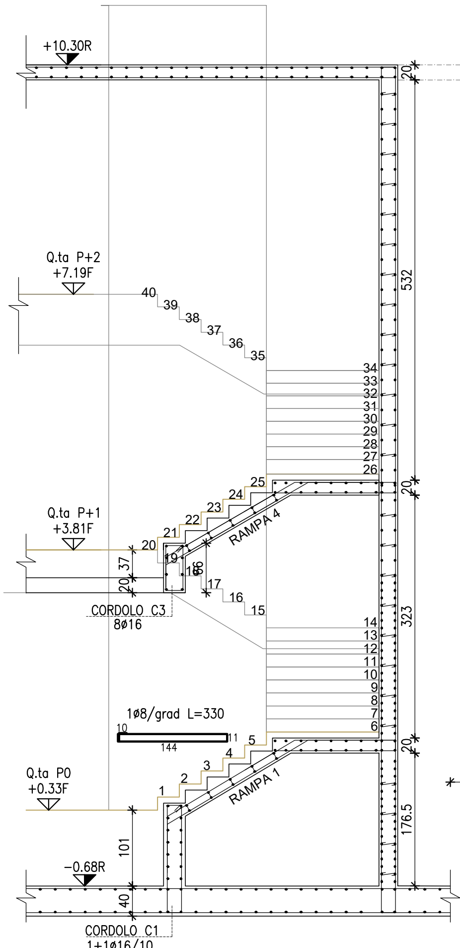
SEZIONE S1 scala 1:50
