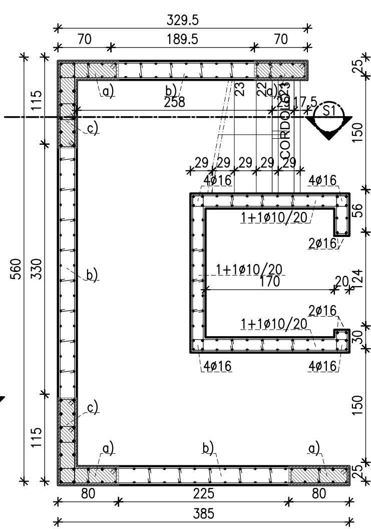
STRALCIO PANTA SECONDO IMPALCATO scala 1:50
