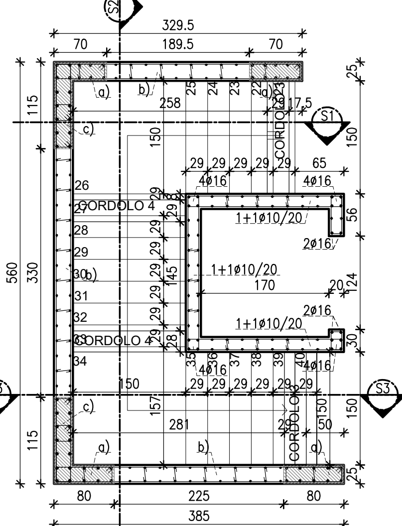
STRALCIO PANTA PRIMO IMPALCATO scala 1:50
