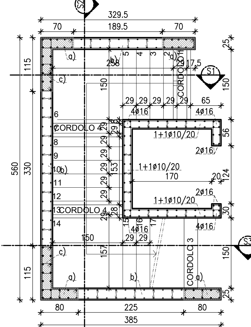
STRALCIO PANTA FONDAZIONI scala 1:50
