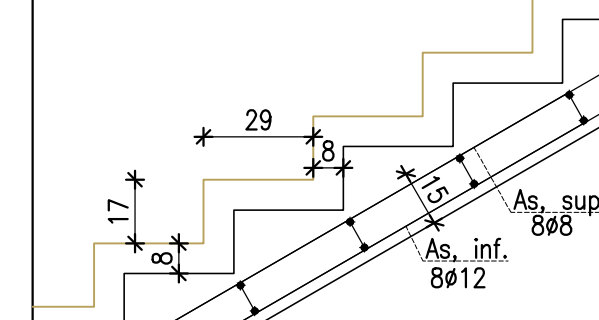
DETTAGLIO GRADINO RAMPA 4-5-6 scala 1:20
