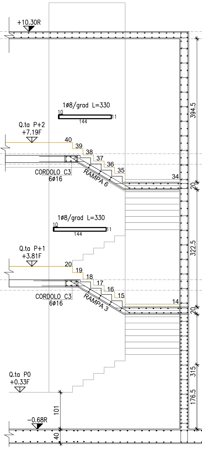
SEZIONE S3 scala 1:50
