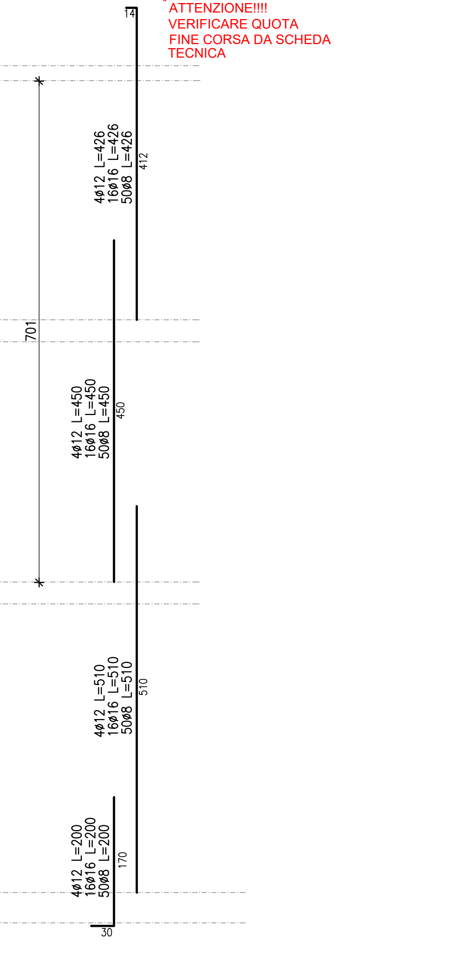
SVILUPPO FERRI VANO ASCENSORE scala 1:50
