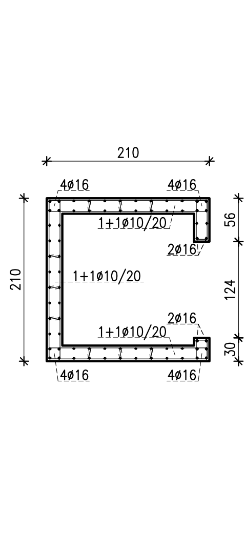
STRALCIO PANTA FUORI CORSA scala 1:50
