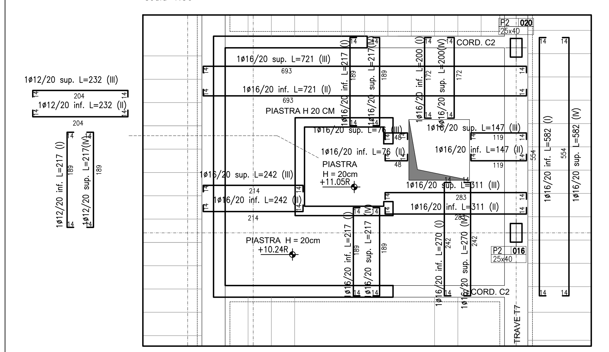
STRALCIO VANO SCA E ASCENSORE -- ARMATURA CORRENTE scala 1:50
